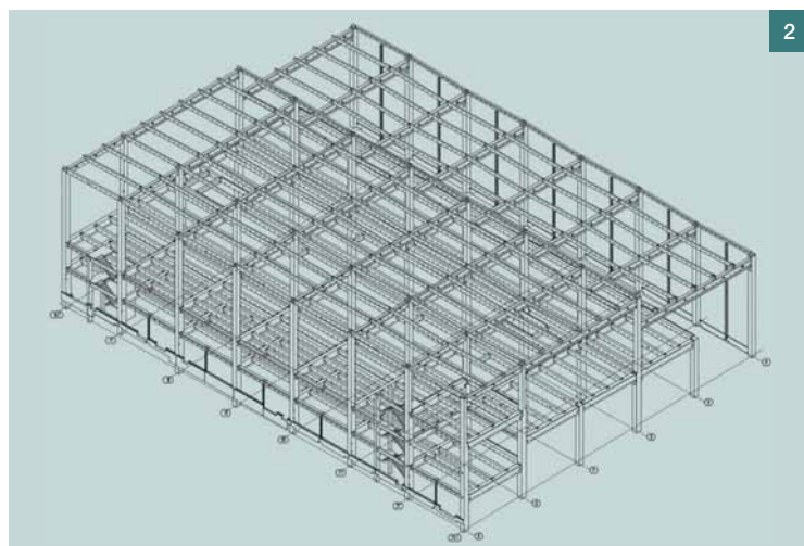
Obr. 1 Celkový model 3D objektu haly 2A lakovna ■ Fig. 1 3D visualisation of the building hall 2A paintshop
