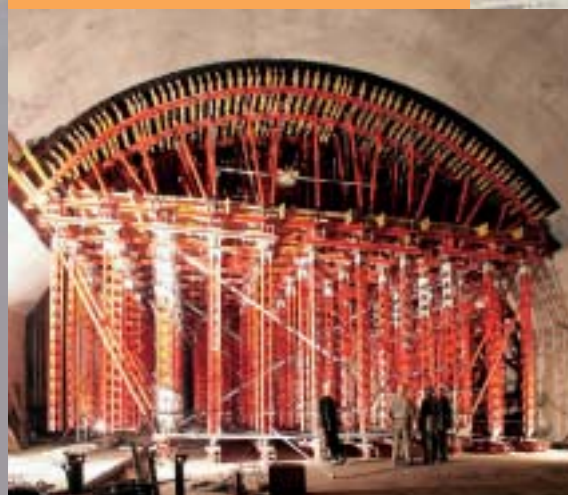
Bednění vrcholu klenby zálivu ZTT Casing of the Vault Top of the West Tunnel Bay
