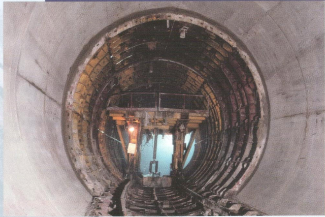
Tunel Mrázovka – kalota rozpletu
